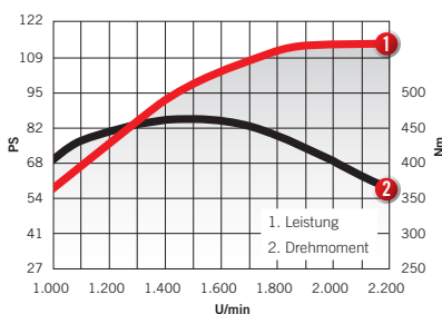
Leistungskurve 4115 Multi:
